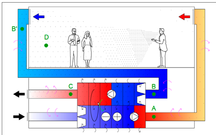
Rys. 2. Potencjalne rozprzestrzenianie się patogenu i miejsca rozważanych lokalizacji dodatkowych urządzeń oczyszczających powietrze (A, B, B', C, D). Fig. 2. Potential spread of the pathogen and locations of additional air purifying devices under consideration (A, B, B', C, D).
