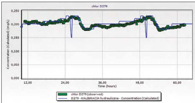
Rys. 8. Porównanie przebiegu zmian stężenia chloru obliczonego i zmierzonego w węźle D279 Fig. 8. Comparison of chlorine concentration changes calculated and observed at node D279
