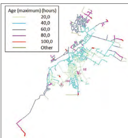
Rys. 10. Wyniki badań symulacyjnych wieku wody Fig. 10. Result of water age simulation
