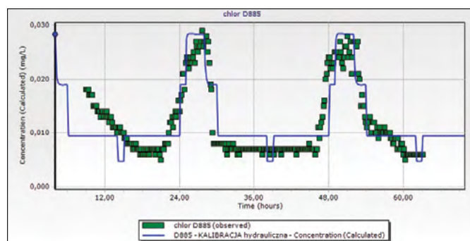
Rys. 6. Porównanie przebiegu zmian stężenia chloru obliczonego i zmierzonego w węźle D885 Fig. 6. Comparison of chlorine concentration changes calculated and observed at node D885
