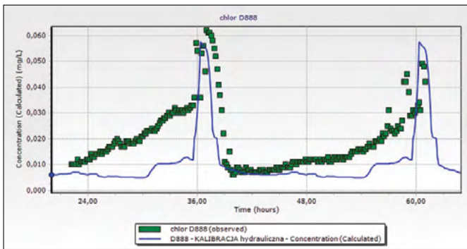
Rys. 7. Porównanie przebiegu zmian stężenia chloru obliczonego i zmierzonego w węźle D888 Fig. 7. Comparison of chlorine concentration changes calculated and observed at node D888
