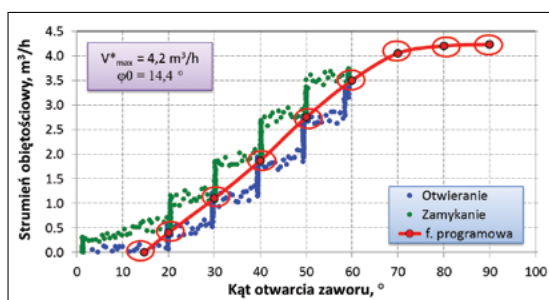
Rys. 8. Charakterystyka zmodyfikowanej procedury OZA z funkcją programową Fig. 8. Characteristics of the modified OZA procedure with program function
