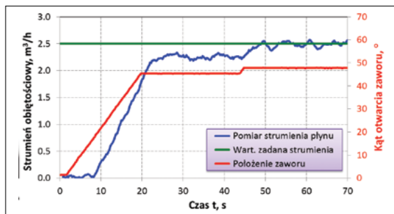
Rys. 9. Charakterystyka sterowania wg funkcji programowej wspomaganie regulacją PID Fig. 9. Control characteristics according to the programme function supported by PID control
