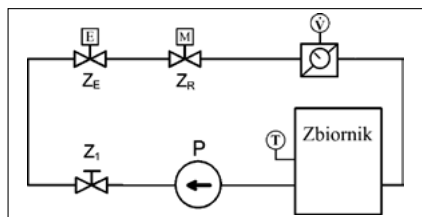
Rys. 2. Schemat stanowiska do badań przepływowych armatury Fig. 2. Diagram of the research stand for the flow armature testing
