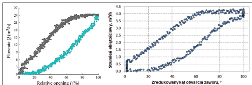
Rys. 1. Strumień płynu w funkcji zredukowanego stopnia otwarcia zaworu: a) wyniki badań wg literatury [1]; b) wyniki badań własnych
